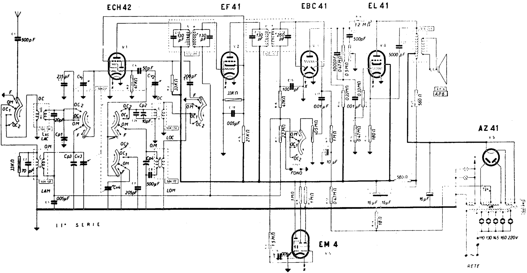
VOCE DEL PADRONE - Mod. 514. Onde medie e due gamme onde corte espanse. Media frequenza 465 kc/s. Potenza di uscita 3,5 watt. Consumo 35 watt (questo è lo schema del mod. 514; lo schema del mod. 594 II a serie differisce solo per il valore di C8 che è di 440 picofarad).
